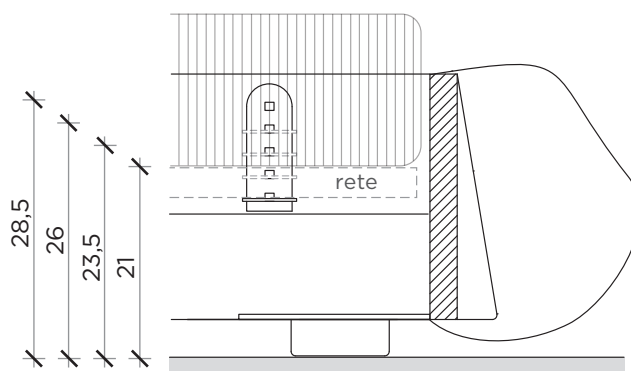
POSSIBILITÀ DI REGOLARE L'ALTEZZA DELLA RETE
