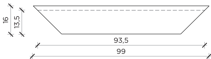
PIANTA | PLAN
