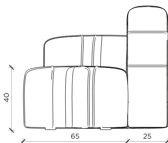
LATO | SIDE
