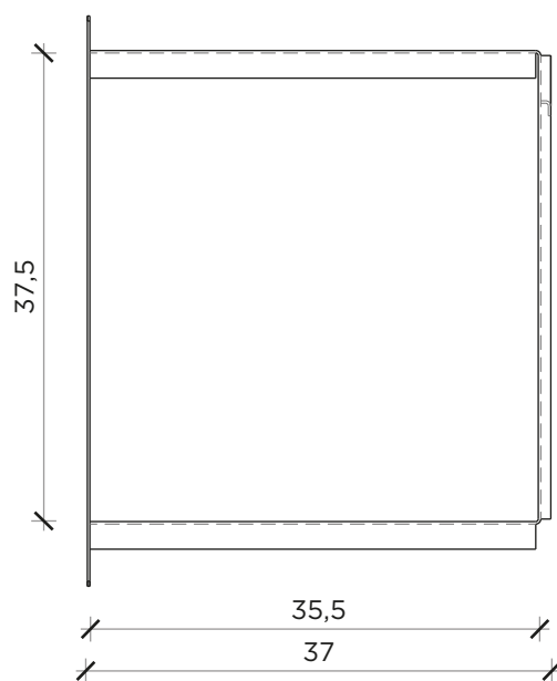
LATO | SIDE
