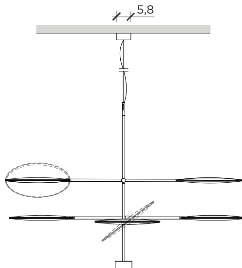
LATO | SIDE
