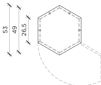
PIANTA | PLAN
