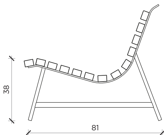
LATO | SIDE
