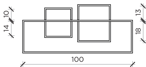
LATO | SIDE
