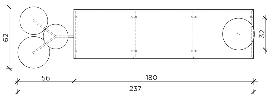
PIANTA | PLAN
