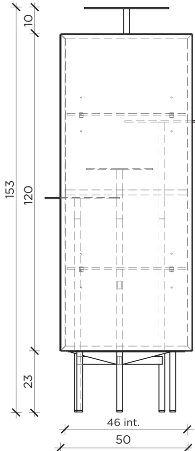
LATO | SIDE
