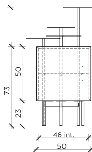
LATO | SIDE
