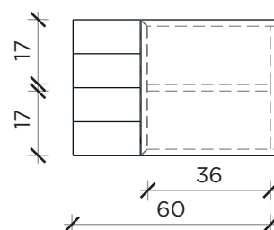
LATO | SIDE
