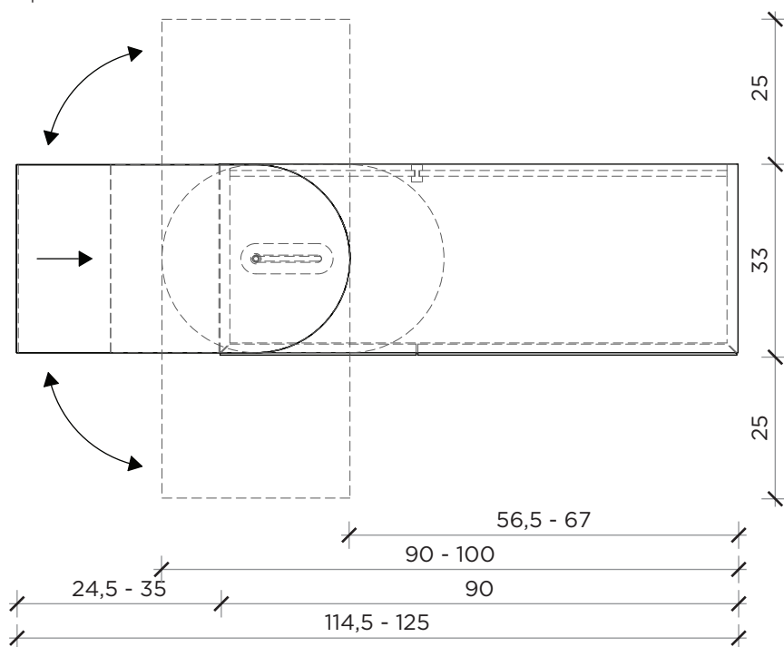
PIANTA | PLAN
