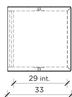
LATO | SIDE
