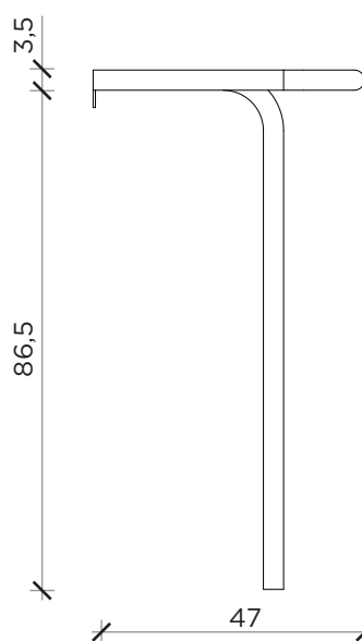
LATO | SIDE
