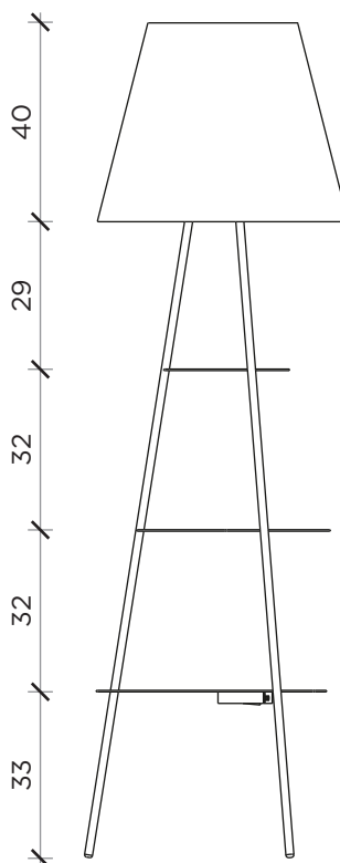
LATO | SIDE
