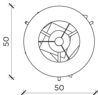
PIANTA | PLAN
