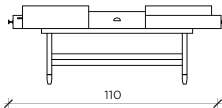
LATO | SIDE
