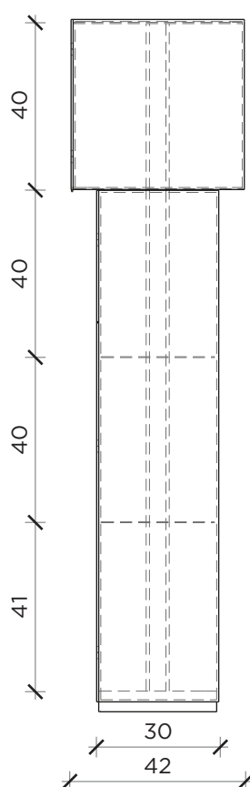
LATO | SIDE
