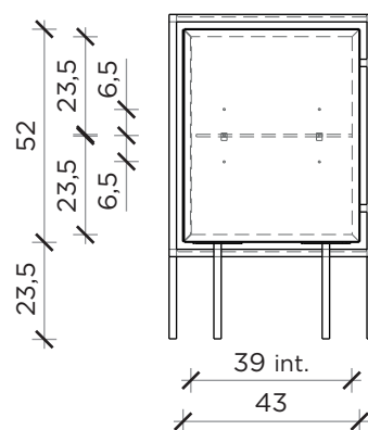
LATO | SIDE
