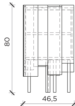
LATO | SIDE
