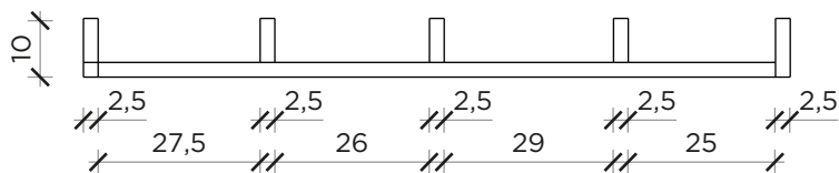
PIANTA | PLAN
