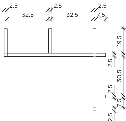
PIANTA | PLAN
