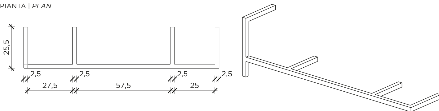
PIANTA | PLAN
