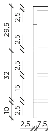
LATO | SIDE
