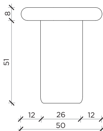
LATO | SIDE
