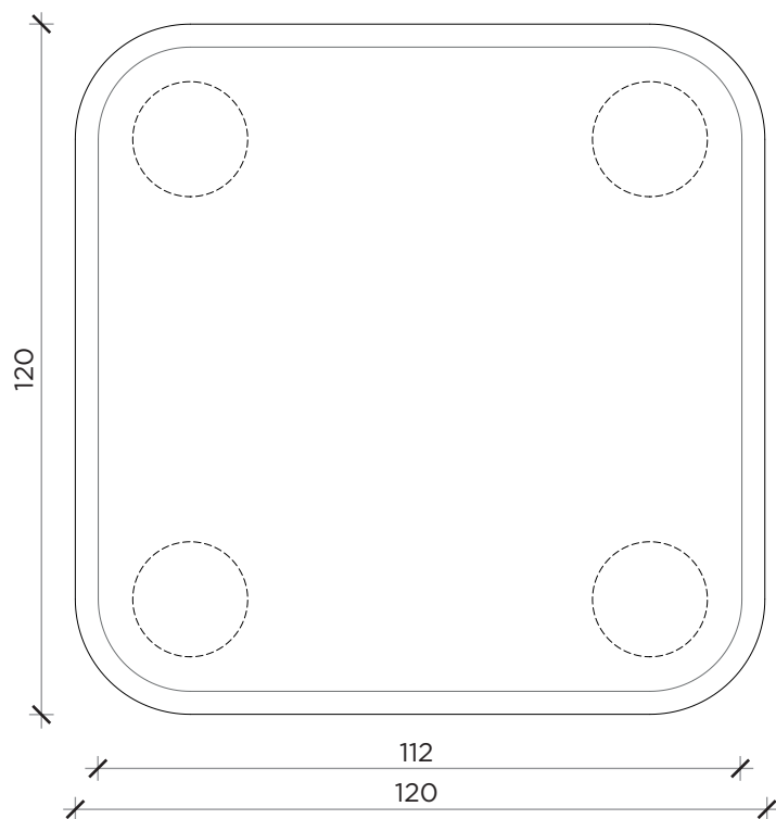
PIANTA | PLAN
