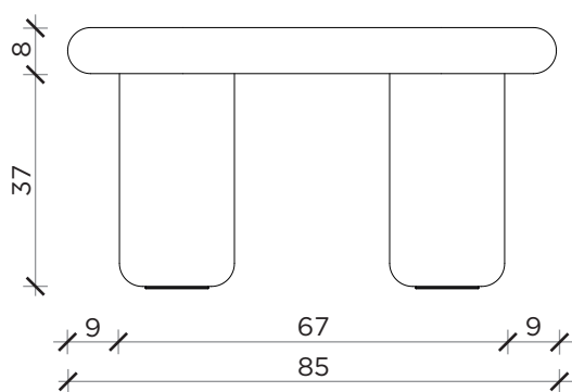
LATO | SIDE
