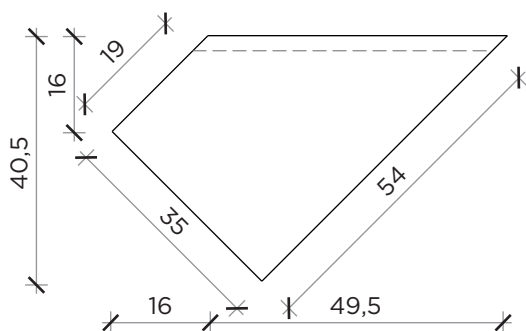
PIANTA | PLAN
