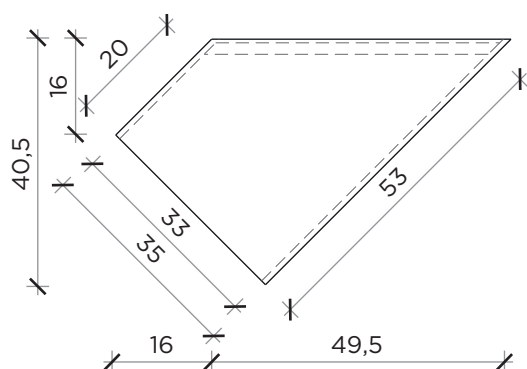
PIANTA | PLAN
